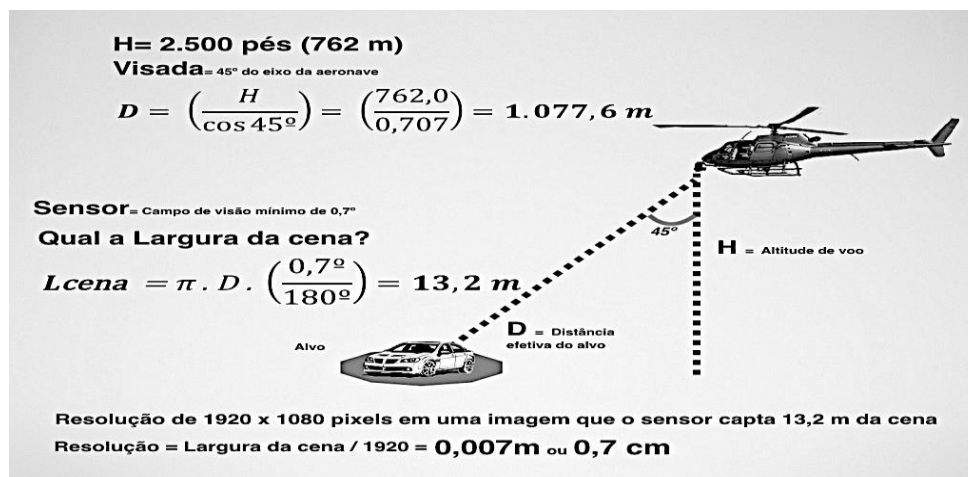
FIGURA 9: LEITURA DE PLACA VEICULAR E RESOLUÇÃO NO SENSOR DE AERONAVES
